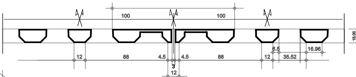
face sup
